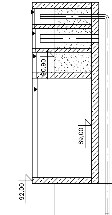
Komora rozdzielacza
